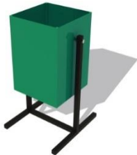
Урна №1. 190x190x380мм Цена – 2400 руб.
