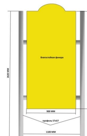
Доска информации №3. Цена – 15 000 руб.
