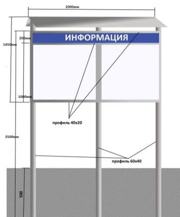
Доска информации №2. Цена – 26 000 руб.
