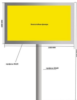
Доска информации №1. Цена – 15 000 руб.
